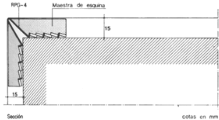
Fig 12. Guardavivos colocado (NTE-RPG 74)
